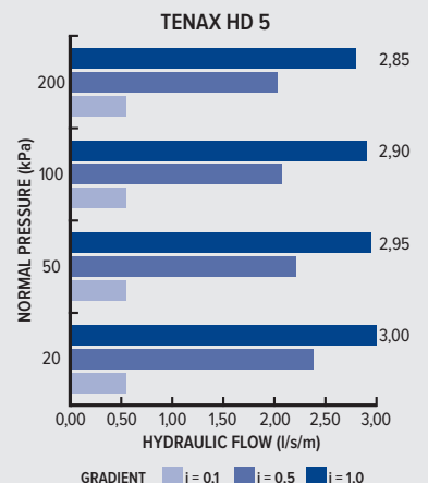
TENAX HD
